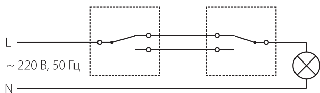
Одноклавишный проходной выключатель
